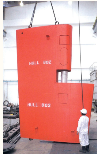
Rudder Blade
